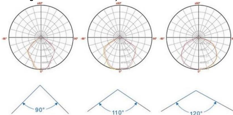
Figura 01: Curva de distribuição de intensidades luminosas
